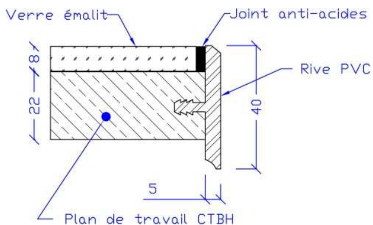
Détail en coupe du plateau
